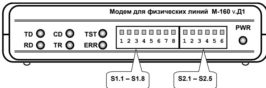
Рис. 3 Передняя панель модема
