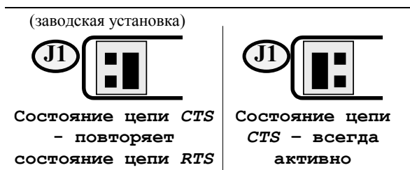
Рис. 6 Положение переключателя на переключателе J1
